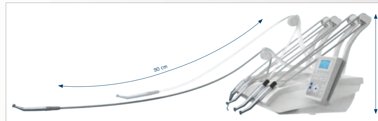
Doskonała ergonomia przy każdym zabiegu: mała wysokość ramion rękawów 45 cm, maksymalna długość wyciągania rękawów instrumentów wynosząca 90 cm.
