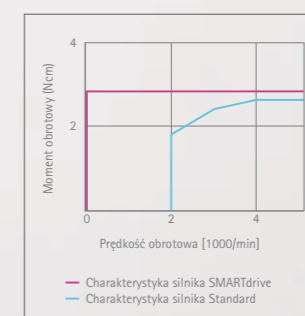
SMARTdrive daje możliwość korzystania z pełnej mocy silnika w poszerzonym przedziale obrotów od 100 do 40 000 obr/min.
