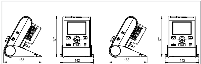
Dimensions FOX
